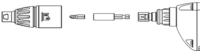
Схема патронник
